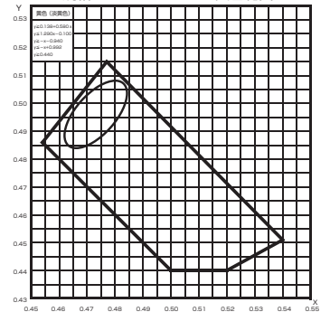
グラフ2 JIS規格D5500-1995 黄色範囲
