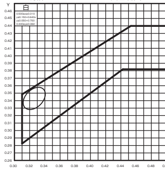
グラフ1 JIS規格D5500-1995 白色範囲
