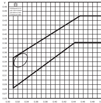
グラフ1 JIS規格D5500-1995 白色範囲
